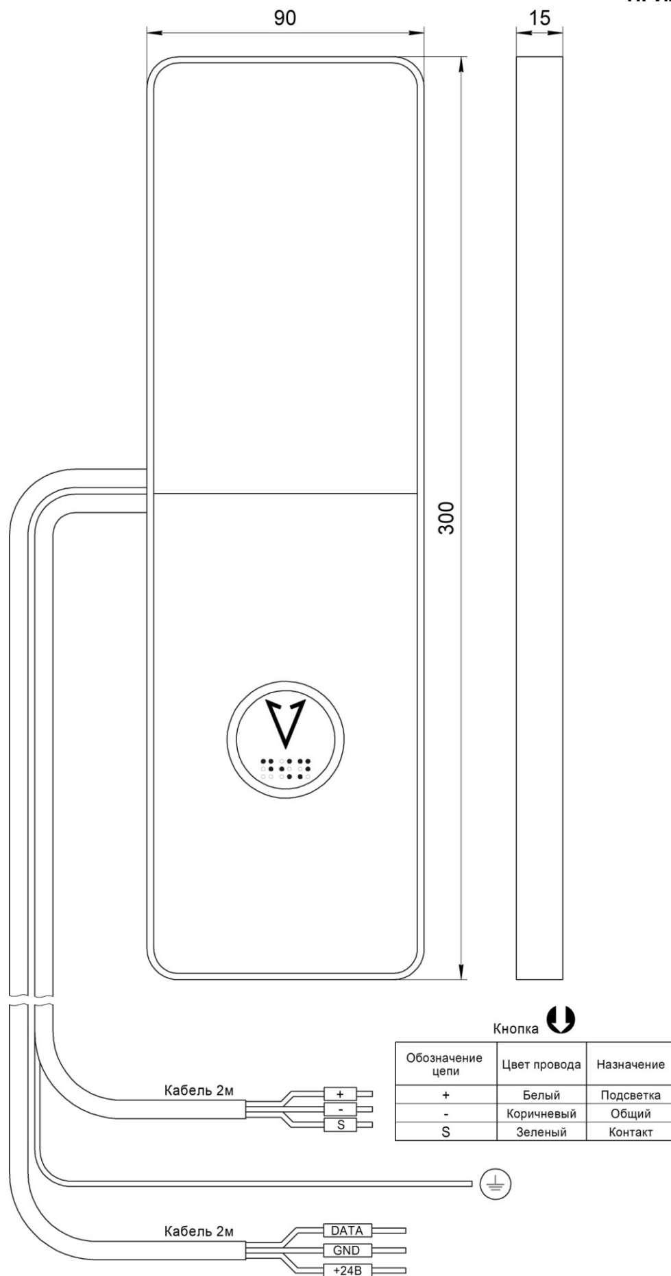
Рис.1 Внешний вид Вызывной пост GOLD (2404) НШЕК.468381.204-01
